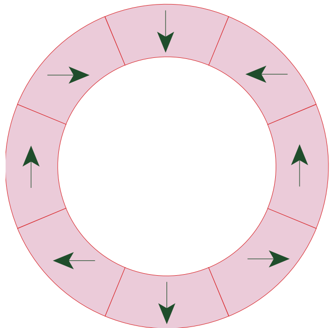
Figure 1a — Halbach Array
